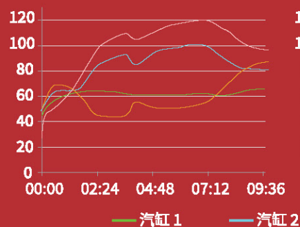
髒污累積後惡化的冷啟動運轉狀態
