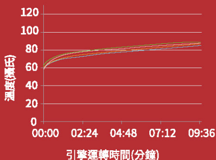
乾淨燃料噴嘴最佳冷啟動運轉狀態
